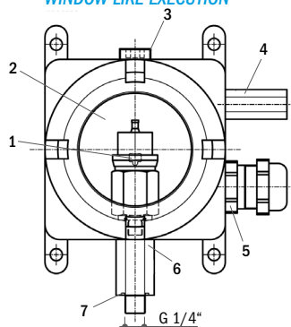
VERSIONE APERTA CON OBLÒ WINDOW LIKE EXECUTION
