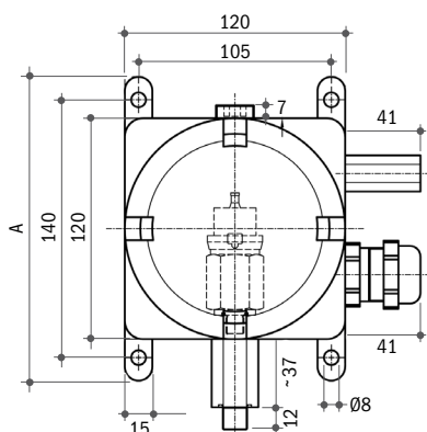
VERSIONE CHIUSA BLIND COVER EXECUTION
